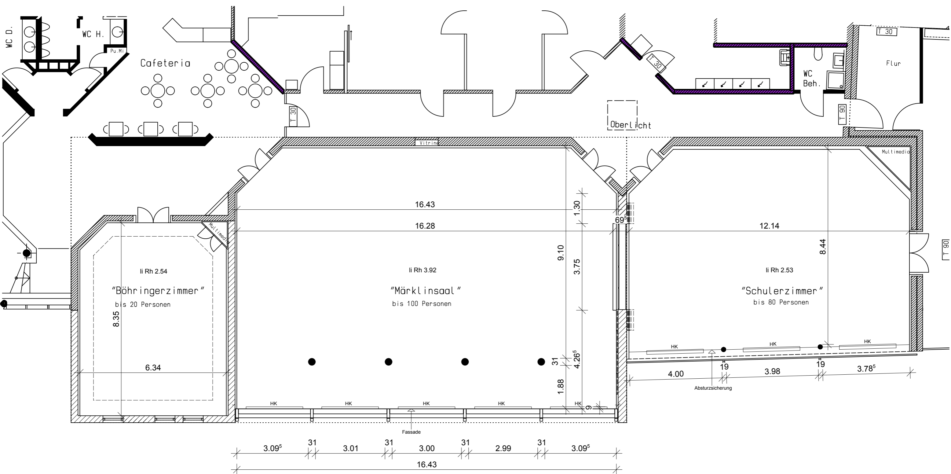
Stadthalle Göppingen Konferenzbereich Teilgrundriss 1.OG M 1:100 FB6/65/6.10.16
